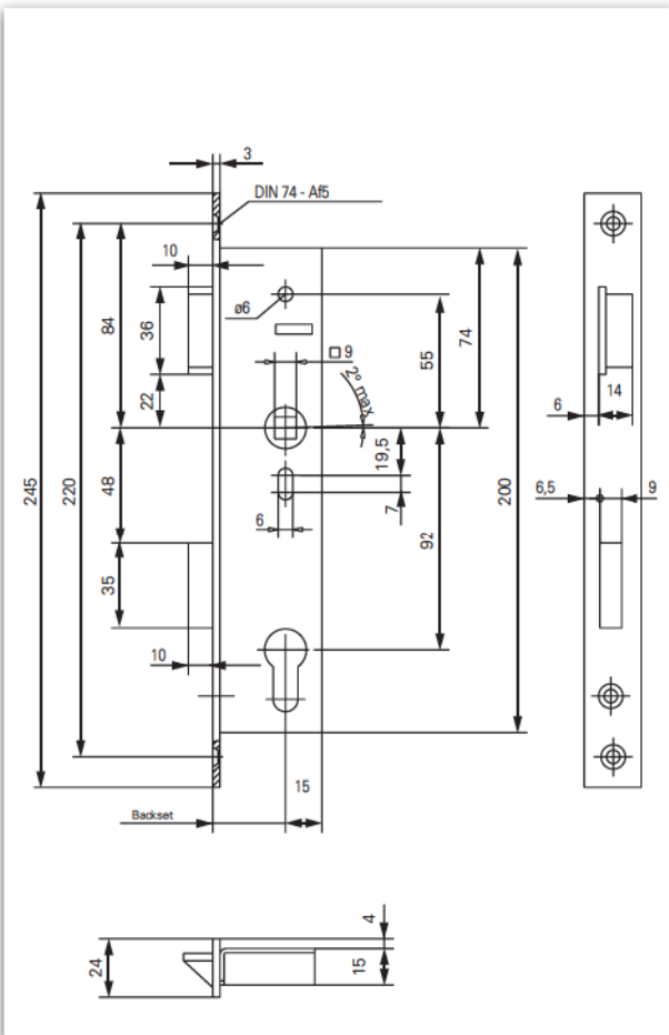
Dimensioning: GBS 71
