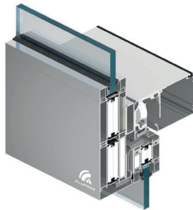
Aluprof MB78 EI DPA Automatic Sliding Door
